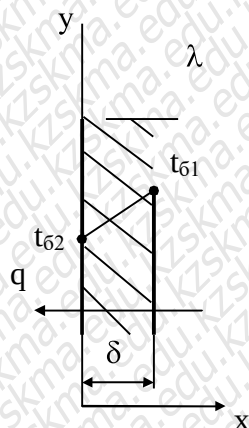
13.1 сурет. Жазық қабырғаның жылуөткізгіштігі
