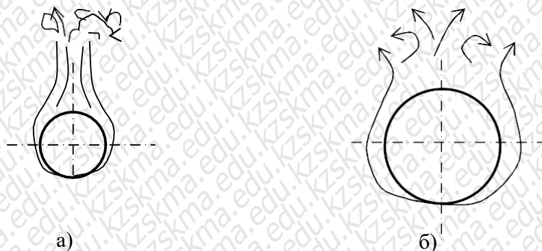
16.6 сурет. Горизонталь құбыр жанындағы ерікті конвекция.
